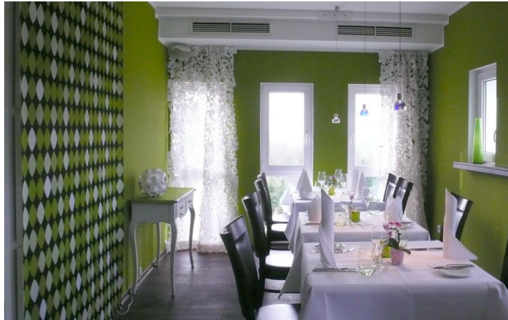
6 Absorptionsplatten ..... unter dem Grafikvorhang (links im Bild).
